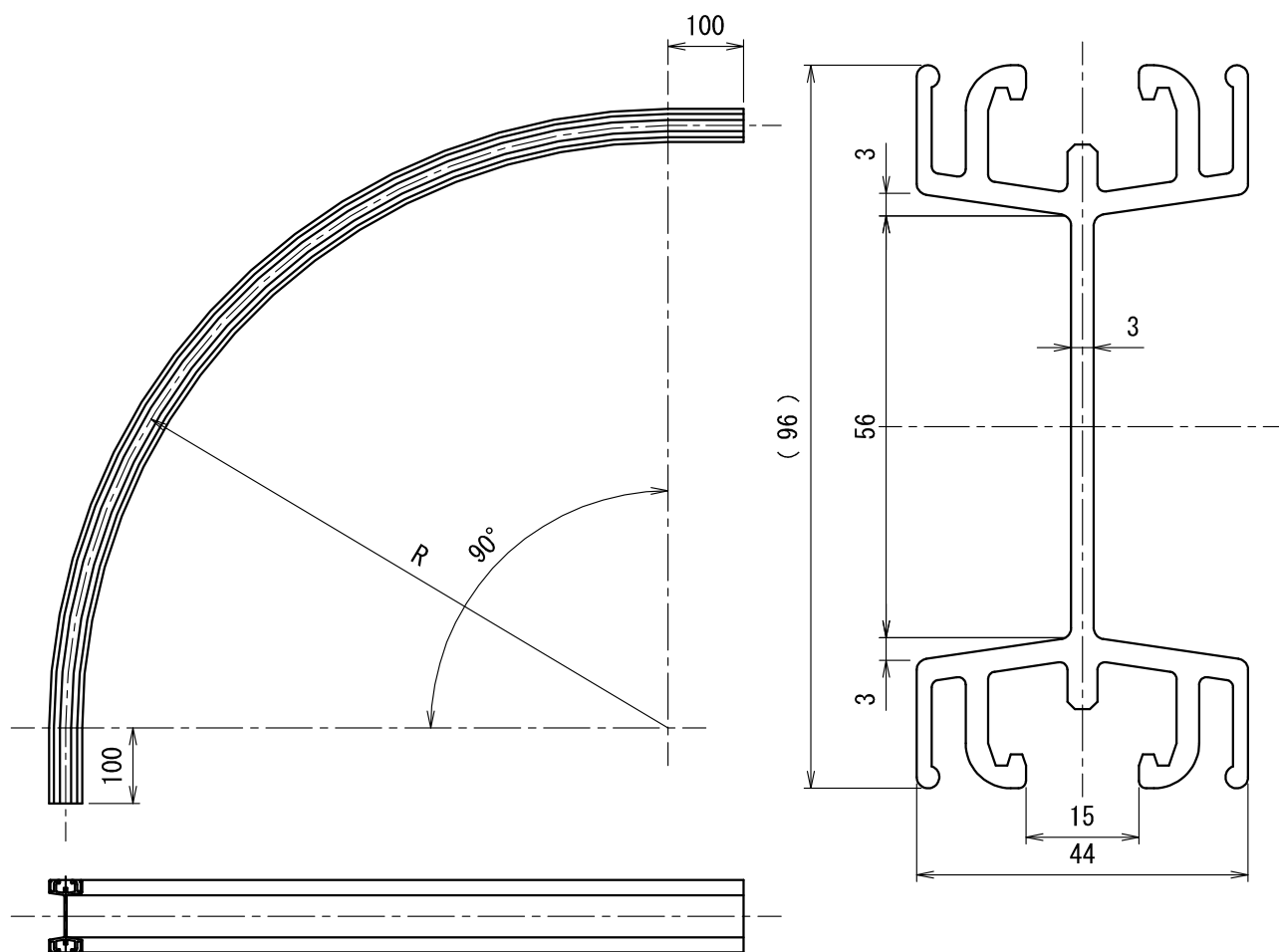
製品断面詳細図(1/1)
